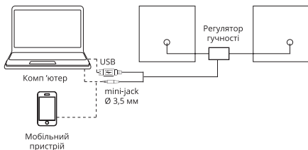
Мал. 1. Схема підключення
