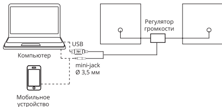
Рис. 1. Схема подключения
