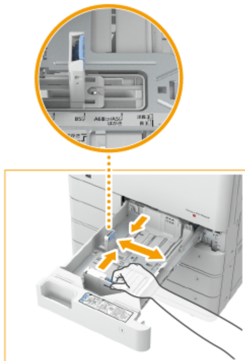
Кассета для бумаги 1
