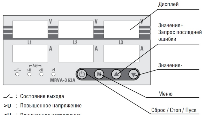
Рис. 5. Дисплей и индикация
