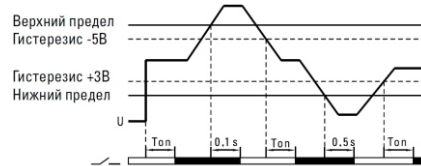
Рис. 1 Диаграмма напряжения реле
