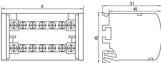
Рисунок 1. Габаритные размеры шин ШНК 2x7 и ШНК 2x15
