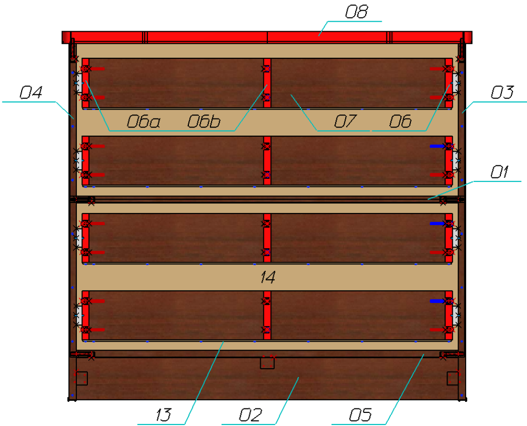
Схема сборки. Комод Лотос.
