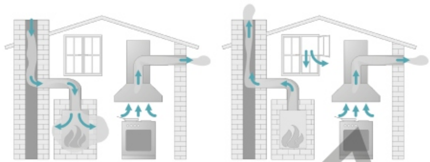
Рис. 3 Одновременная эксплуатация вытяжки и устройства горения
