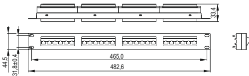
Рисунок/Figure 2 – PP24-1UC5EU-D05D
