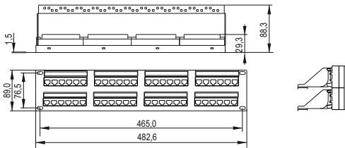
Рисунок/Figure 8 – PP48-2UC5EU-D05-1
