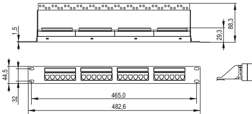
Рисунок/Figure 7 – PP24-1UC5EU-D05-1
