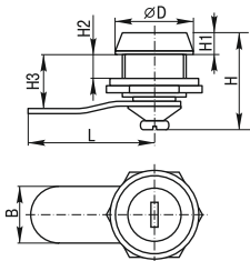
Рисунок 2. Замок 18-18/34
