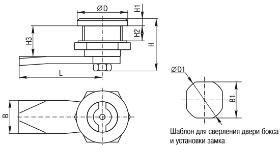
Рисунок 5. Замок-защёлка с пластмассовым ключом IP54 22-17/46
