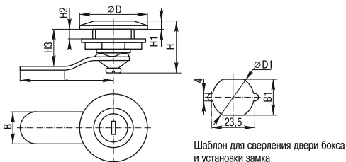
Рисунок 1. Замки 20-22/40, 20-22/45
