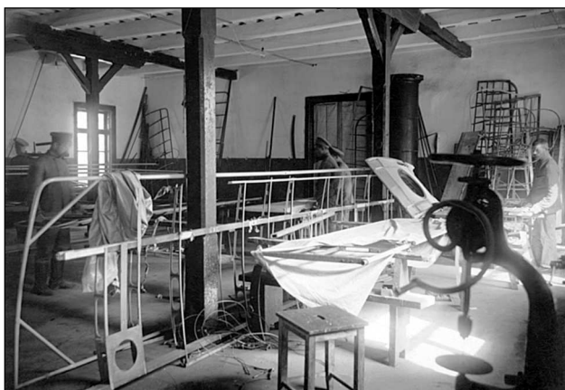
Сборка деревянных крыльев и раскрой полотняной обшивки
