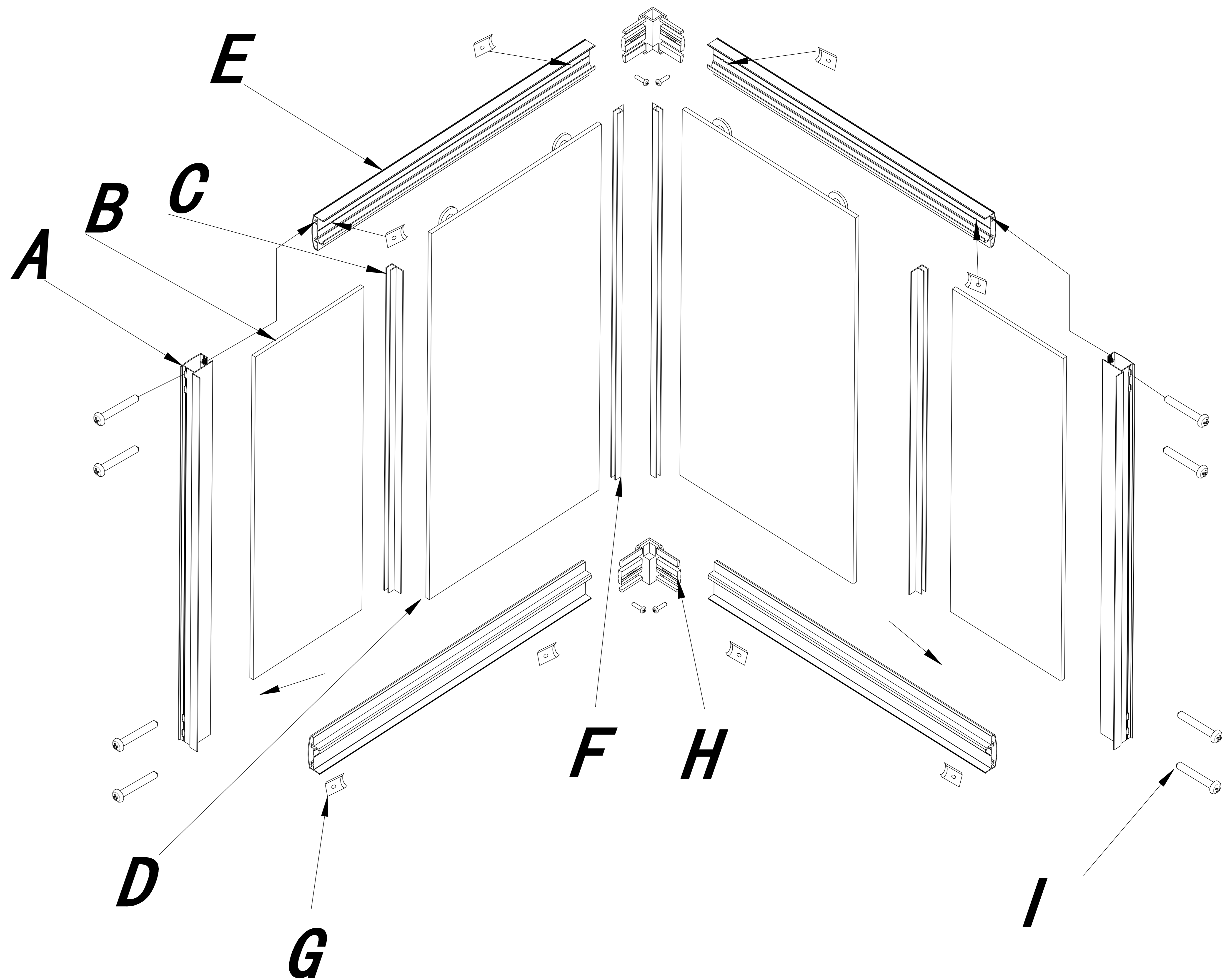
Демонтажная схема
