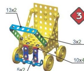
коляска
