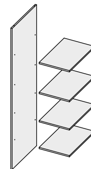
Комплект полок с перегородкой ТД-307.07.02-01
