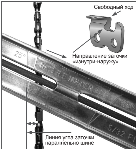
Рис.22 Определение угла заточки
