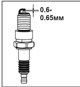
Рис.19 Свеча зажигания
