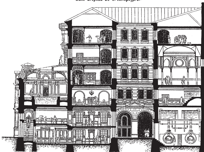
Иллюстрация 3. Егоровская баня в Санкт-Петербурге, построенная в конце XIX века. На 5 этажах располагались мужское и женское отделения, комнаты, предназначенные для приема пищи, чтения, парикмахерская, бассейн и, конечно, парилки. (Строитель. 1896. № 1. С. 53–54.)
