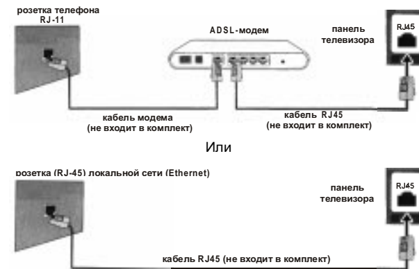
Рисунок 6 – Проводное подключение
