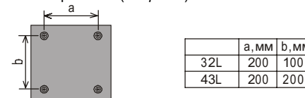
Рисунок 4 – Размеры для выбора настенного кронштейна
