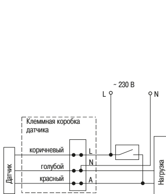
Рисунок 27 – Схема режима постоянного включения нагрузки
