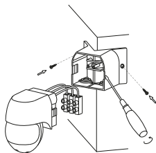
Рисунок 18 – Монтаж ДД 015, ДД 016
