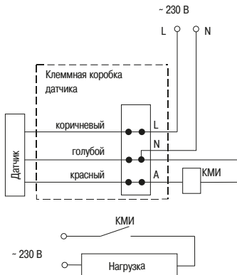
Рисунок 28 – Схема подключения датчика с контактором КМИ
