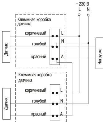
Рисунок 26 – Схема параллельного подключения датчиков
