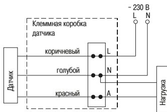
Рисунок 24 – Схема подключения датчиков типов ДД 022, ДД 023
