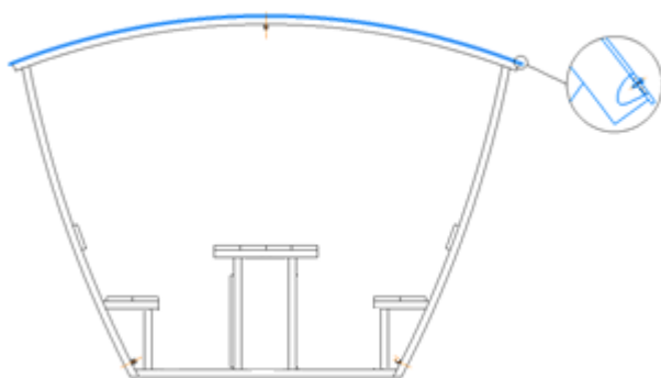
Схема №4 – Крепление поликарбоната на беседки
