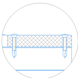
Схема №3 (а, б) – Расположение и крепление досок
