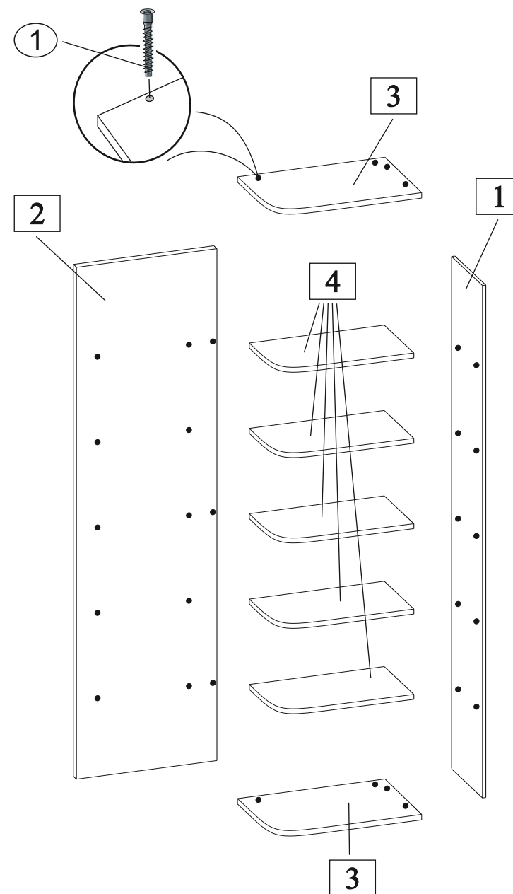
( рис. №1 ) СХЕМА СБОРКИ ЭЛЕМЕНТА
