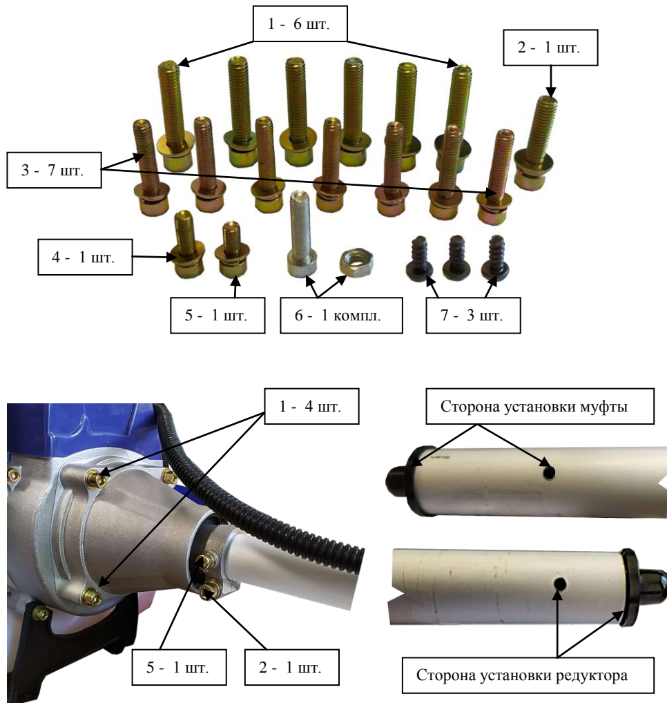
Комплект крепежа и пояснительная схема его установки
