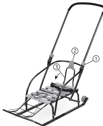
рис. 1 Санки Nikki 2 в разложенном виде
