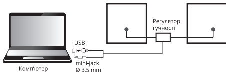
Мал. 1. Схема підключення
