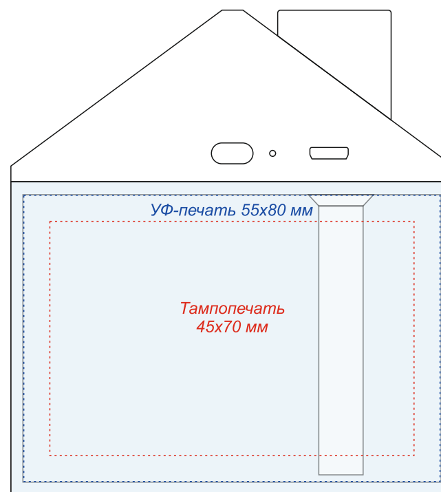
вид сзади
