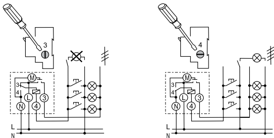
Рисунок 3. Электрические схемы подключения таймера
