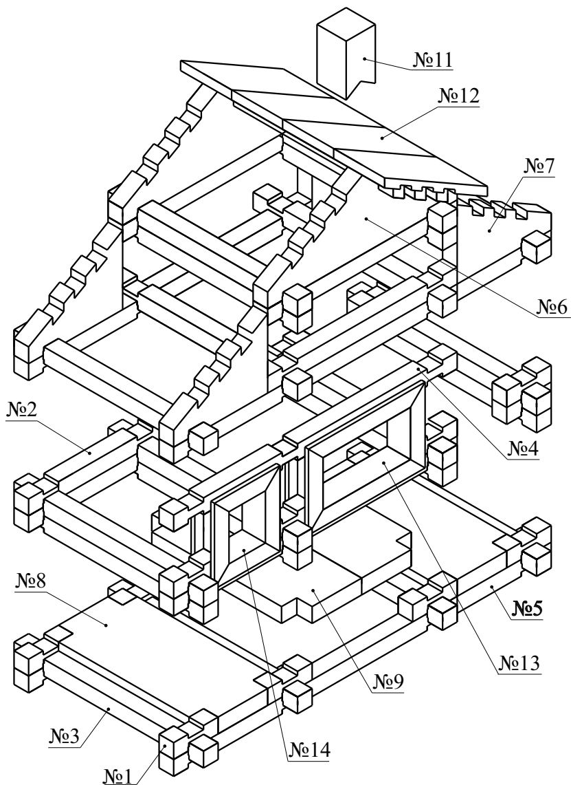
Последовательность сборки домика
