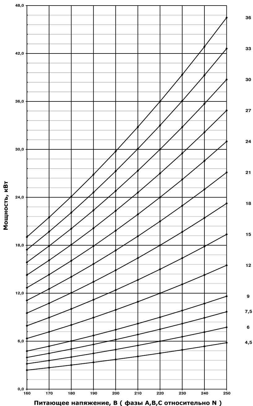
Рис.8 График изменения мощности миникотельной в зависимости от питающего напряжения.
