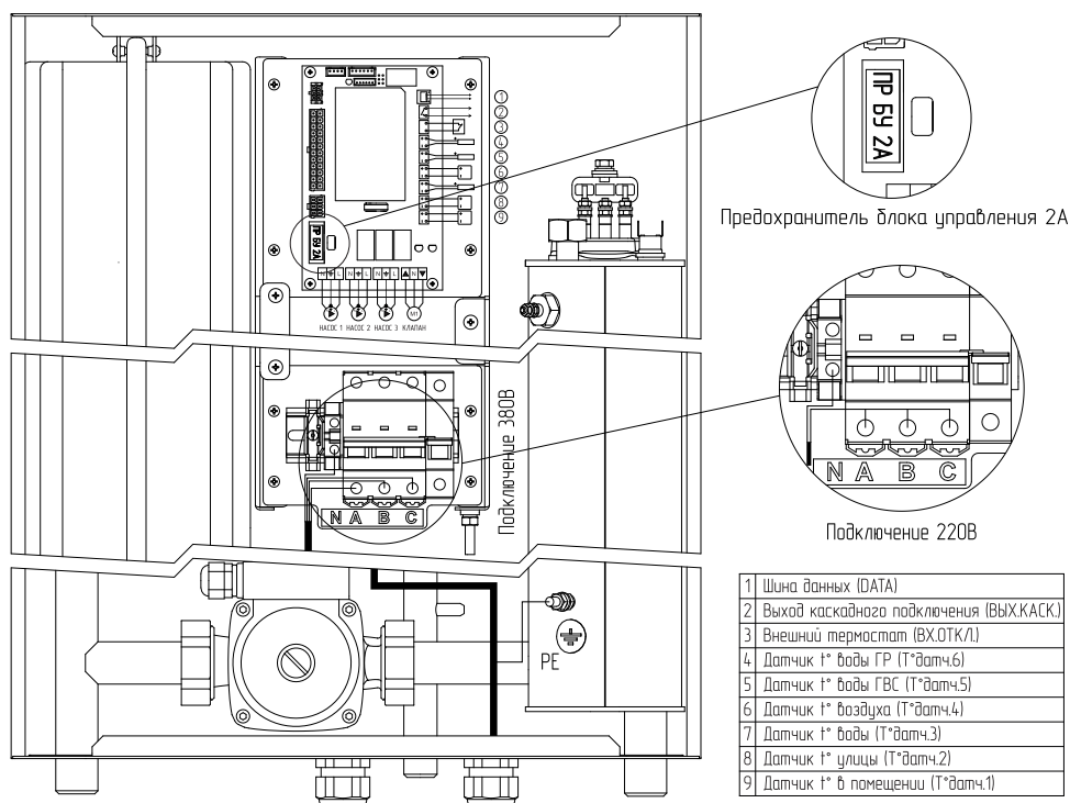
Рис.3 Схема подключения миникотельной.
