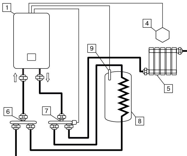
Рис.6 Упрощённая схема подключения миникотельной в режиме «Отопление-ГВС».
