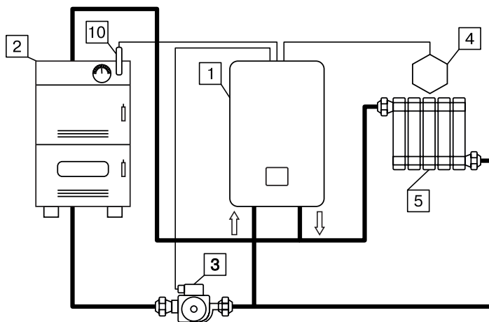
Рис.7 Упрощенная схема подключения миникотельной в режиме вспомогательной.
