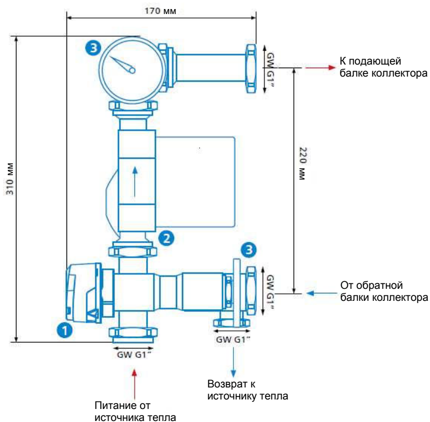
Рис.2 Описание элементов и размеров модуля BRU
