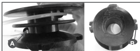
Рис.14 Установка корда
