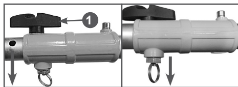
Рис. 3 Установка нижней части штанги
