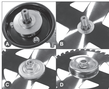
Рис. 5 Установка ножа
