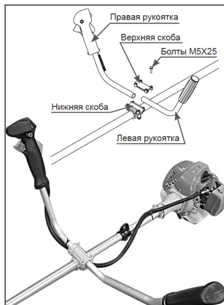
Рис. 4 Установка рабочей рукоятки
