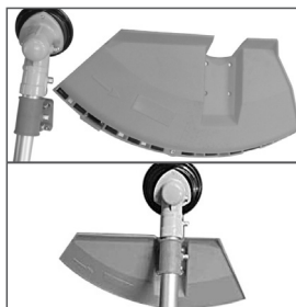
Рис. 2 Установка защитного кожуха
