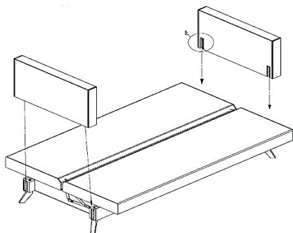
соединитель на подлокотнике
