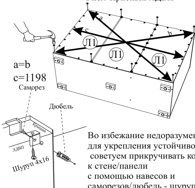
Рис.7 Прибивка ЛДВП
