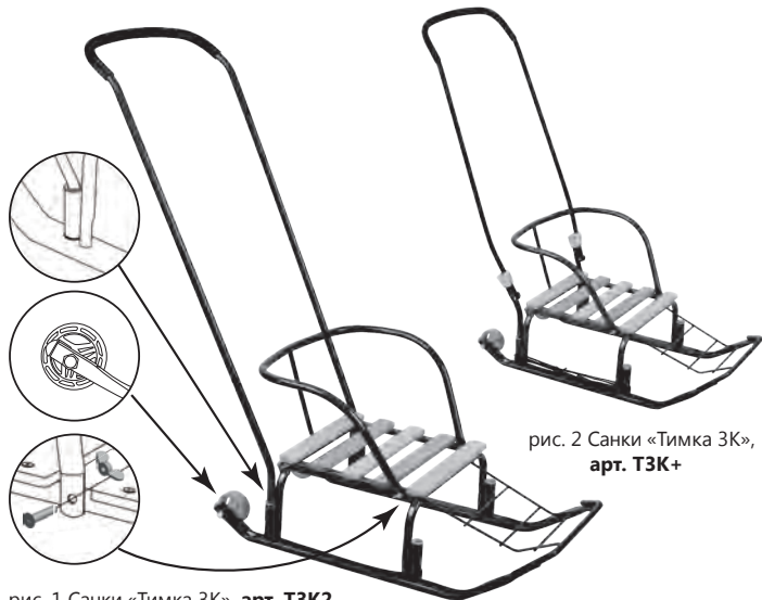
рис. 1 Санки «Тимка 3К», арт. Т3К2
