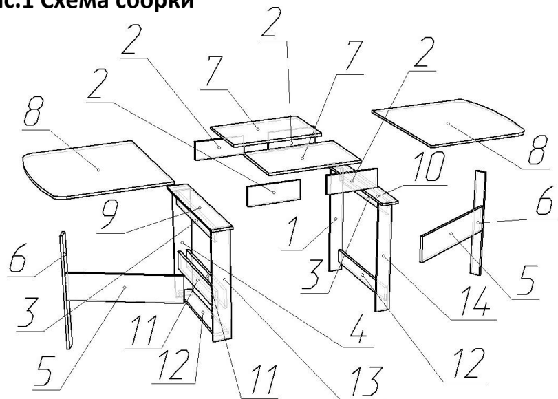
Рис.1 Схема сборки
