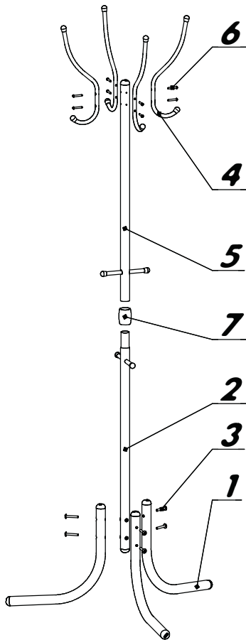
Рис. 1 Схема сборки
