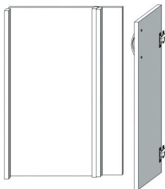
Рисунок 3. Крепление соединительных планок
