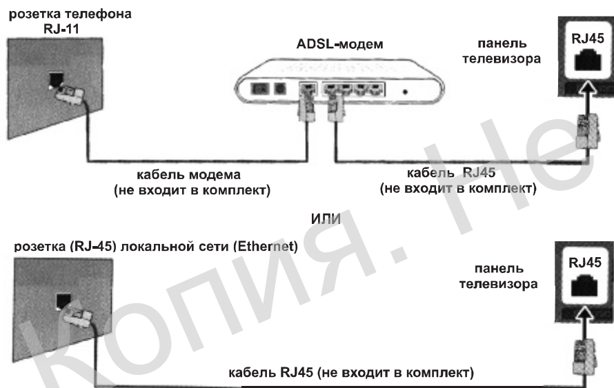
Рисунок 6 – Проводное подключение
