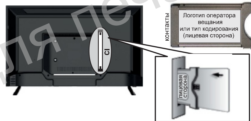
Рисунок 5 – Установка СА-модуля
