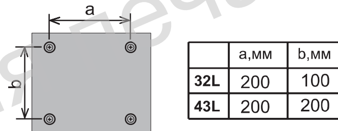
Рисунок 4 – Размеры для выбора настенного кронштейна
