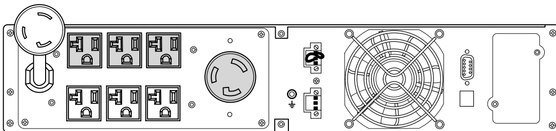
Рисунок 35. Модель PW9130L2000R-XL2U
