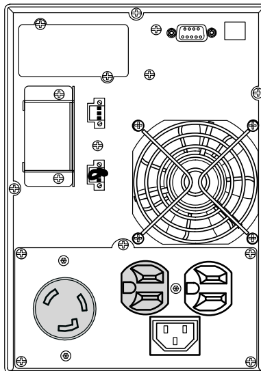
Рисунок 48. Модель PW9130G1000T-XL
