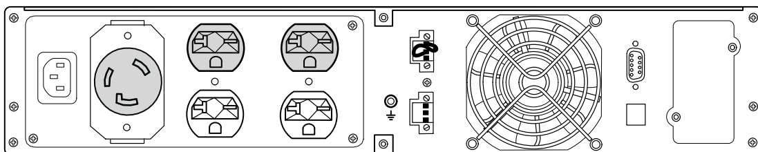
Рисунок 36. Модель PW9130G2000R-XL2U
