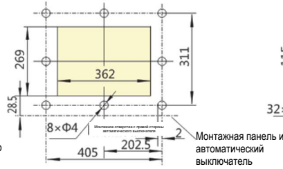
Рисунок 15. NA1-3200X стационарный тип
