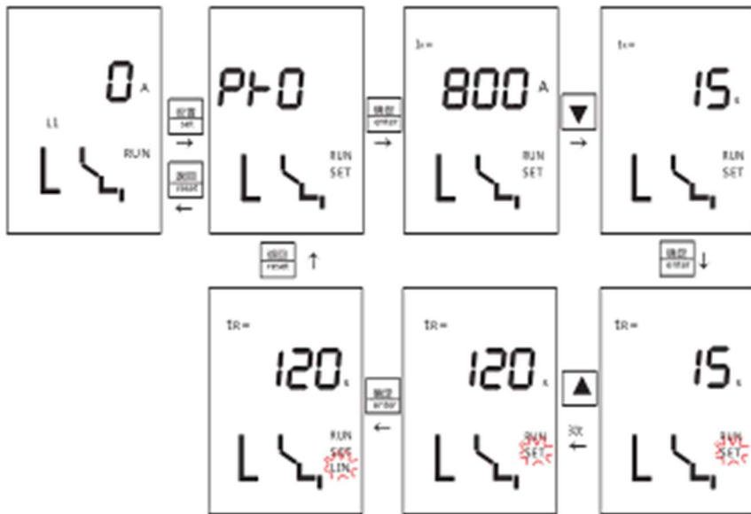
Рисунок 68. Изменение значения времени длительной задержки
