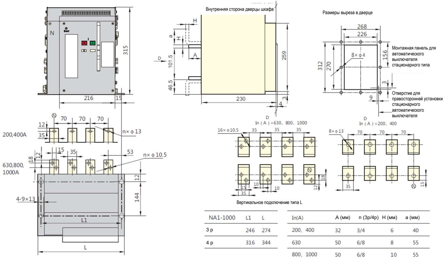
Рисунок 6 NA1-1000X стационарный тип
