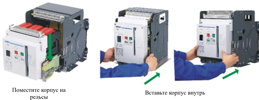
Рисунок 23. Установка корпуса в посадочное место корзины
