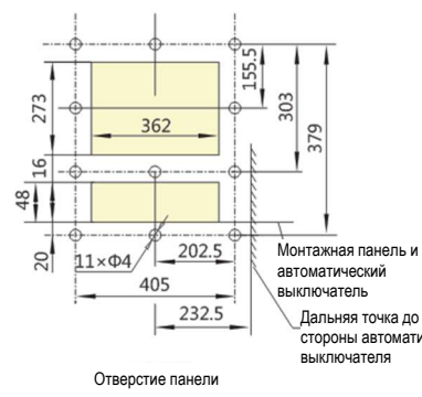
Рисунок 12. NA1-3200X выдвижной тип
