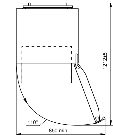
2-Сүрөт – Муздаткыч (Устүнөн көрүнүшү)
