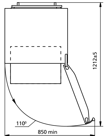
Малюнок 2 – Холодильник (вигляд зверху)
