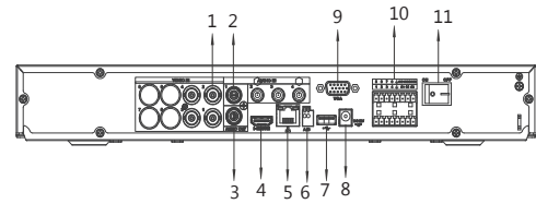
DHI-XVR5204A-S2
