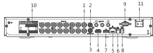
DHI-XVR5216A-S2
