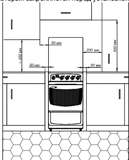
Рисунок 5 – Схема установки плиты
