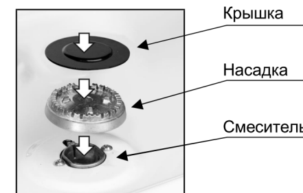
Рисунок 8 – Установка горелки
