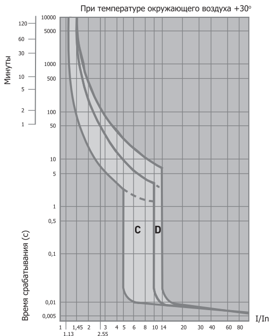
Рис. 1 Время-токовые характеристики выключателей BA 47-100
