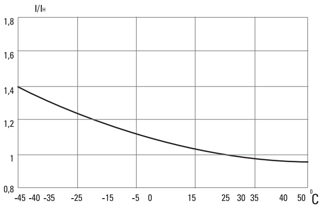
Рис. 2 Температурный коэффициент
