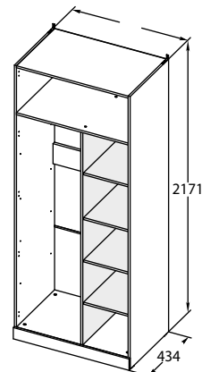
Каркас шкафа для одежды ТД-307.07.22
