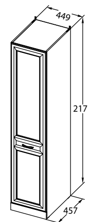
Шкаф для белья ПМ-307.21.00.000
