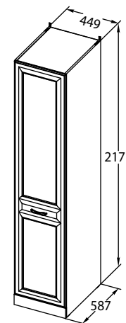
Шкаф для белья ПМ-307.07.00.000
