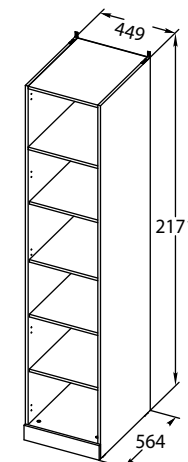
Каркас шкафа для белья ТД-307.07.01
