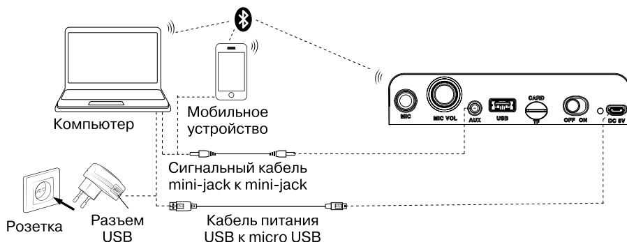
Рис. 3. Схема подключения
