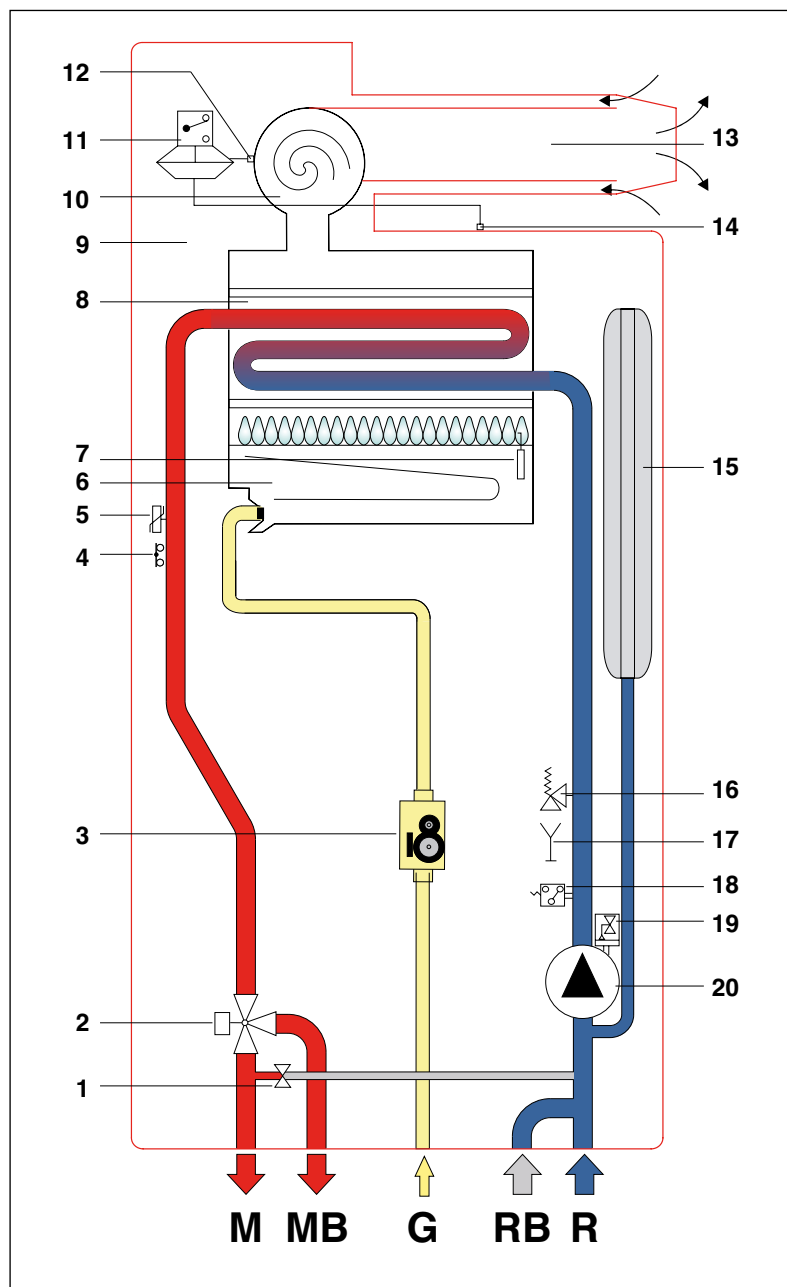
Рис. 8 Гидравлические схемы - RBTF5
