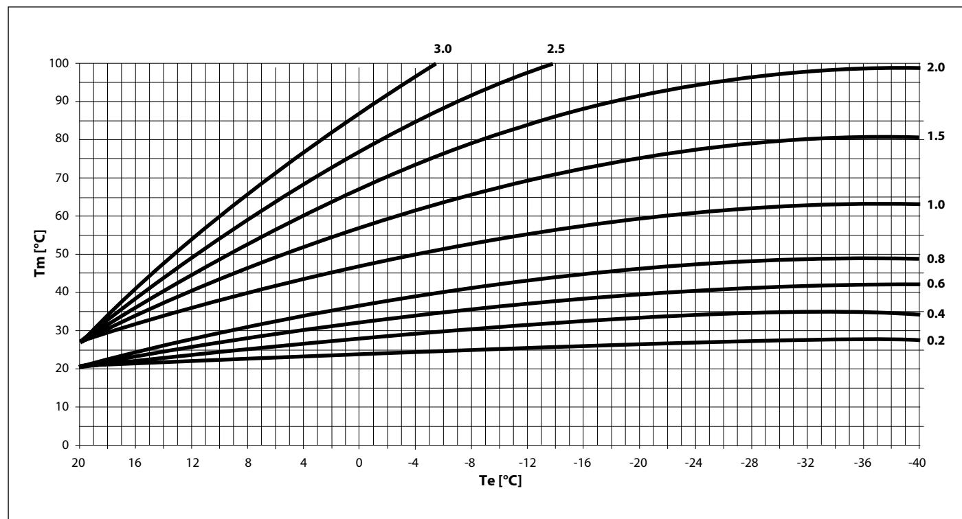
Рис. 16 Температурные кривые
