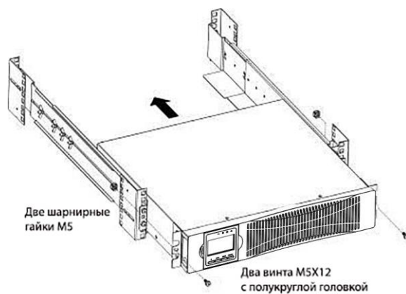
Рис. 4 Фиксация блока ИБП
