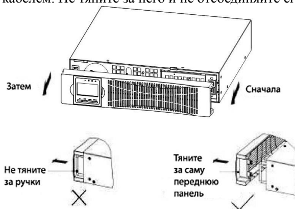
Рис. 5 Снятие передней крышки блока АКБ
