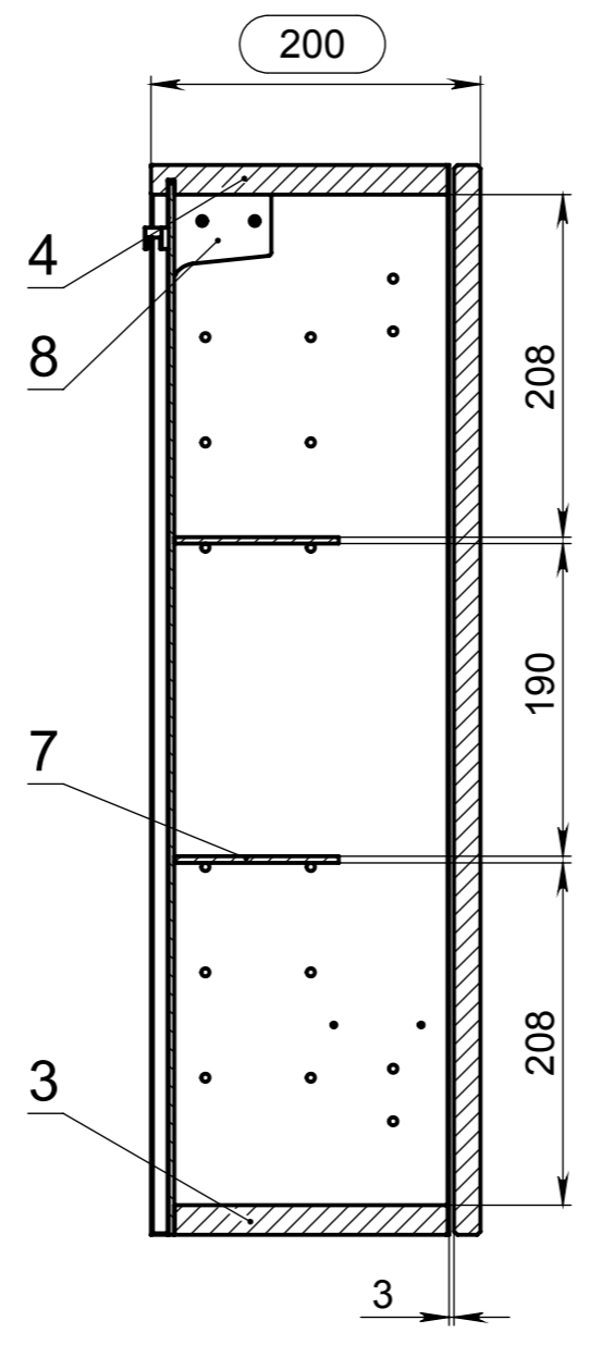
B-B (1 : 5)
