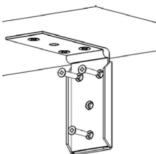
Схема установки спинок
