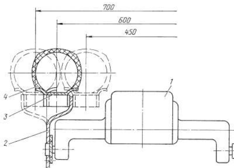
Рисунок 21 – Схема регулирования колеи мотоблока
