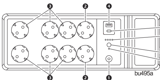
Верхняя панель
